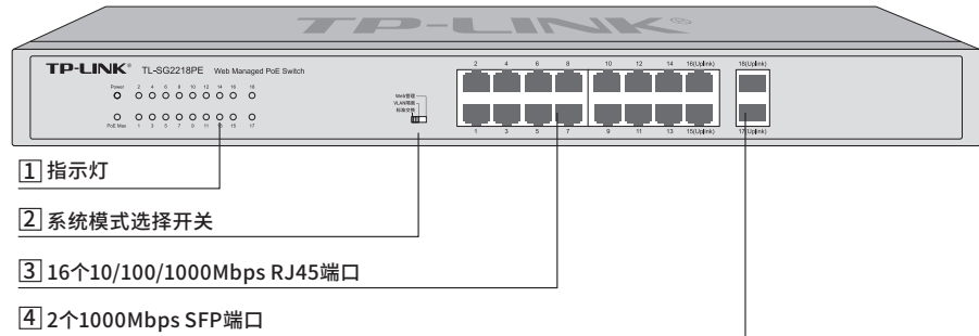
图1-12 TL-SG2218PE前面板示意图
